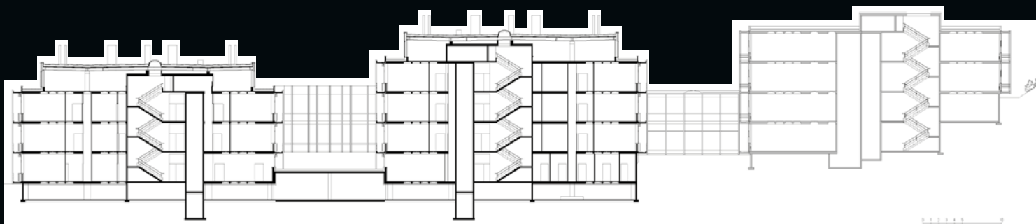
Coupe bâtiment C - D - F
