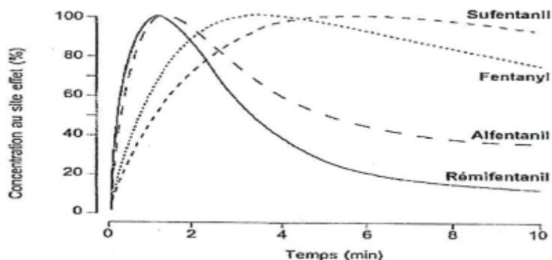
Figure M1 : Graphique représentant la concentration au site d'action en fonction du temps de 4 stupéfiants, exprimée en pourcentage (d'après Shauffer et Varvel)
